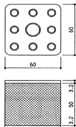
緩衝材(クッションゴム)
