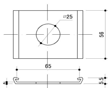
根太パット(塩化ビニル)
