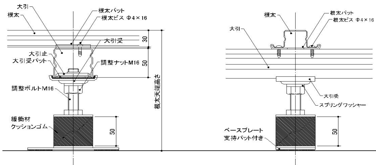
支持脚(一般・端部)
