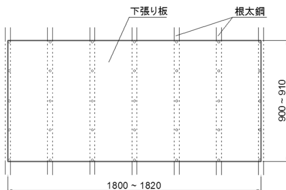
張り込み 留め付け図 - 1
