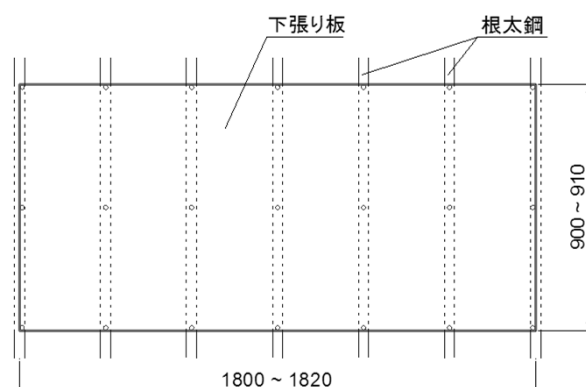
張り込み 留め付け図 - 2
