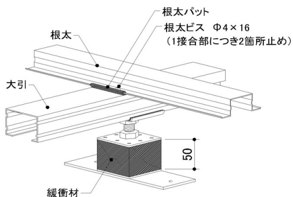
床構成材姿図
