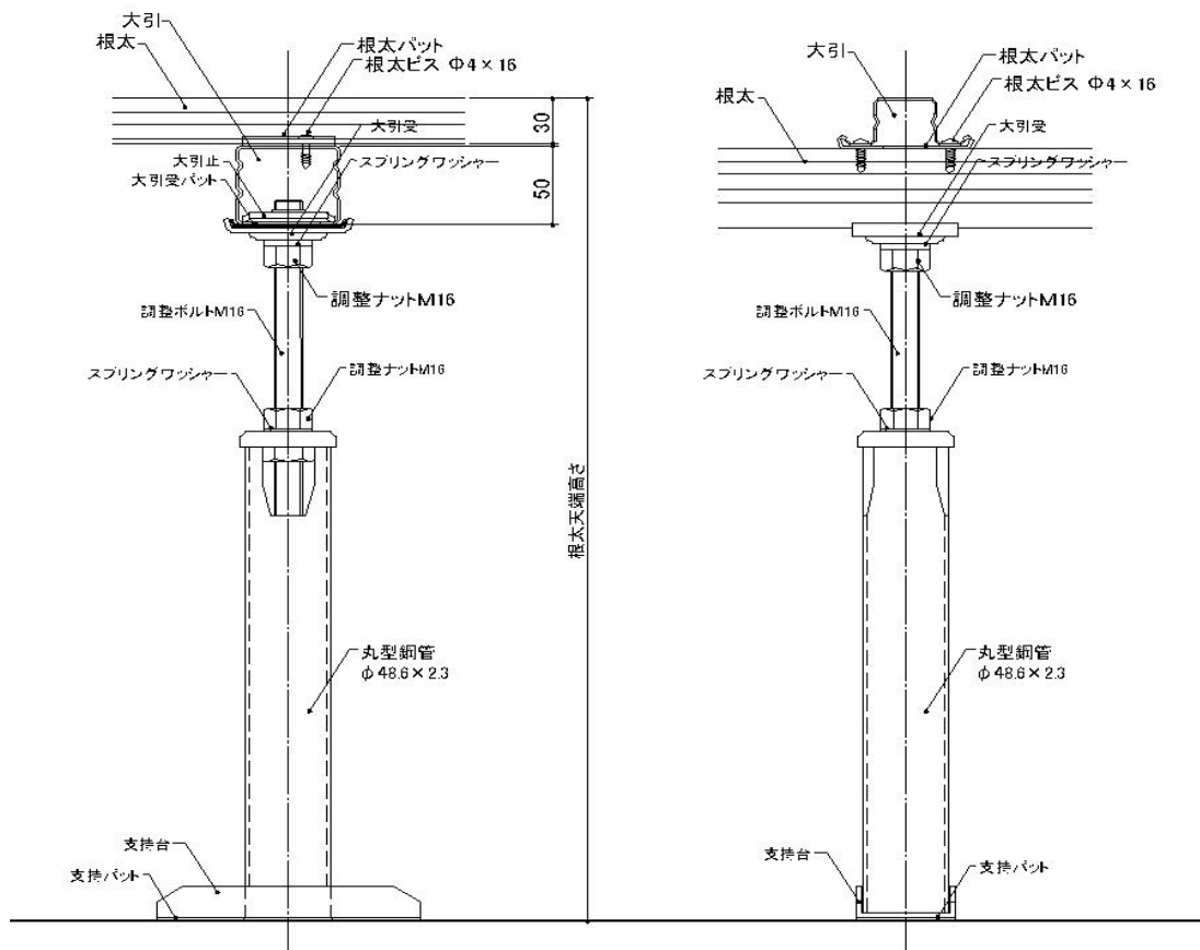
一般支持脚
