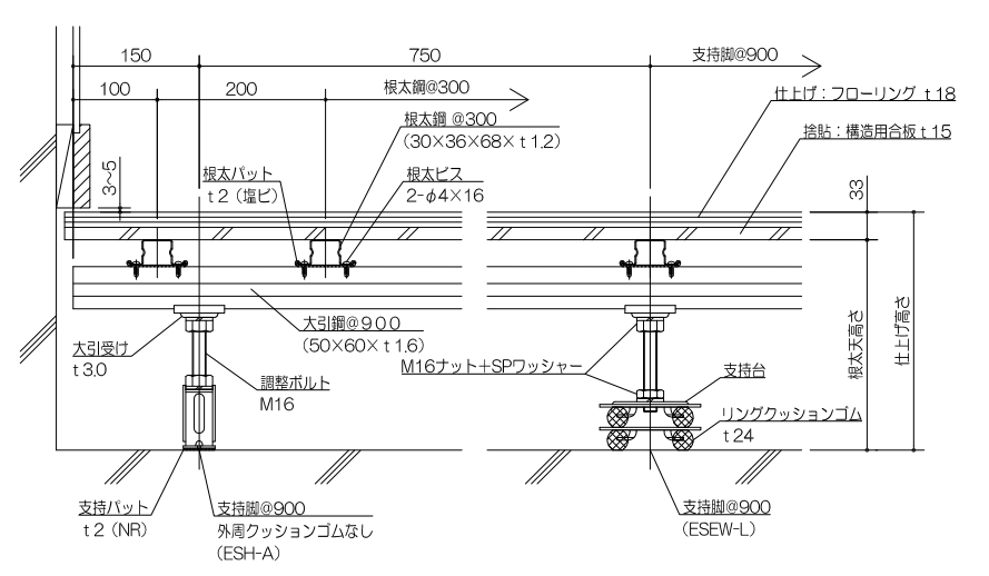
大引方向断面図
