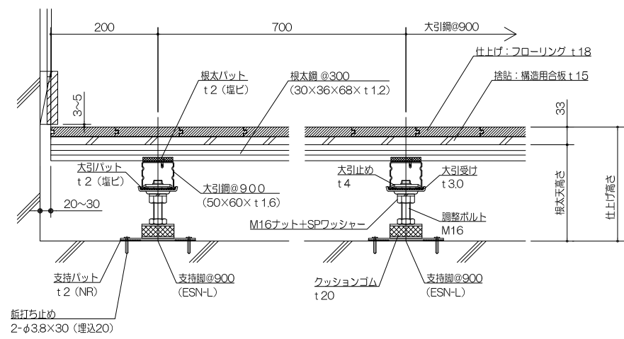
根太方向断面図
