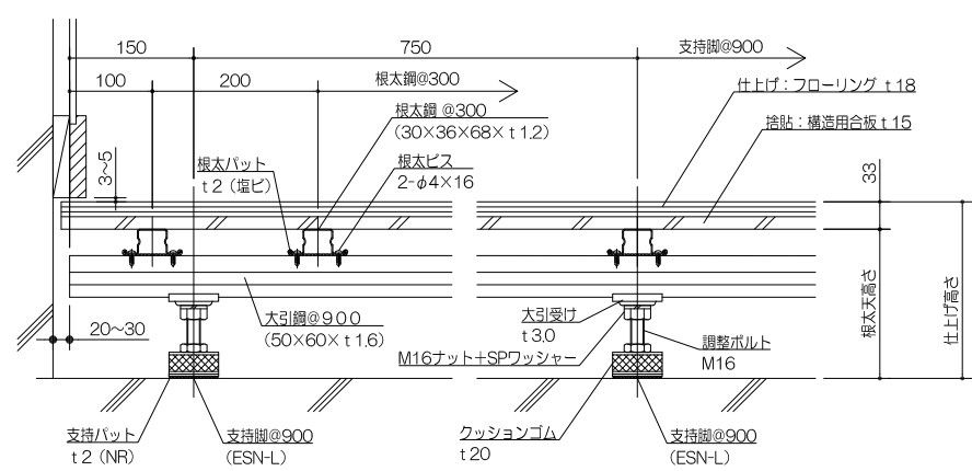
大引方向断面図
