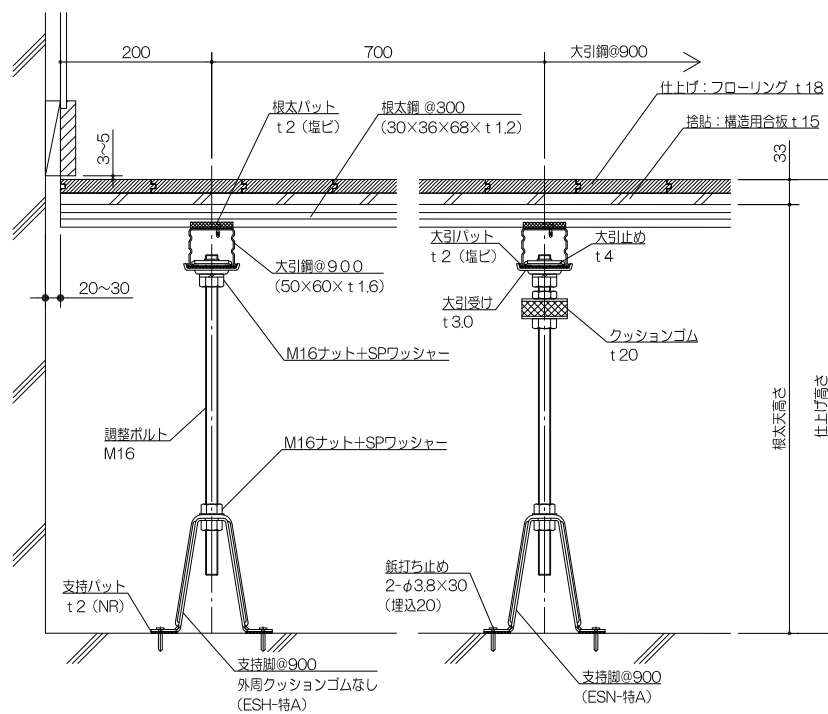
根太方向断面図
