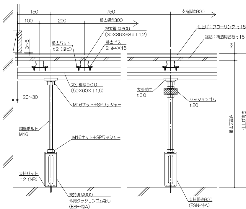
大引方向断面図
