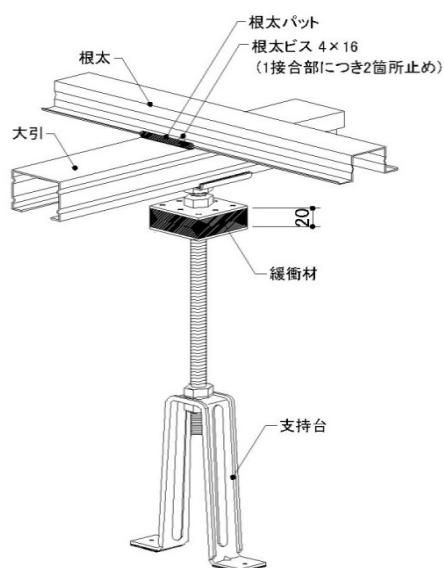
床組構成材姿図
