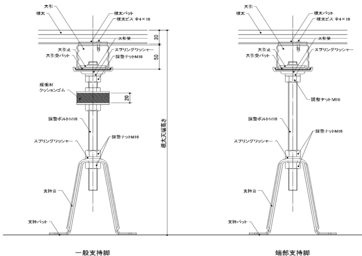
床組構成材姿図
